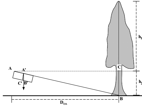
Figura 4.4: Funcionamento da prancheta dendrométrica quando é realizada uma visada da base da árvore.
