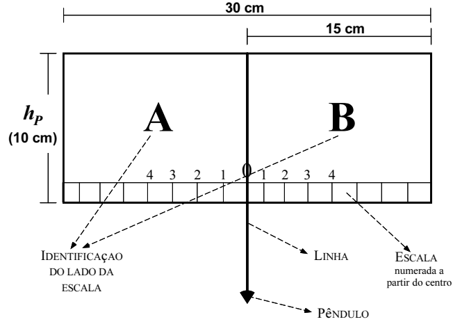
Figura 4.2: Estrutura da prancheta dendrométrica. Material para construção: uma tábua de 30 \times 10 cm, a escala em papel milimetrado e o pêndulo formado de linha e peso.
