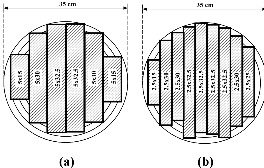
Figura 5.9: Volume útil para serraria considerando tamanho de peças específicos. Em (a) as peças tem espessura constante de 2 cm, enquanto que em (b) a espessura é de 1.5 cm. A largura das peças é variável de modo a aumentar o aproveitamento da tora, já o comprimento das peças é definido pelo comprimento da tora.
