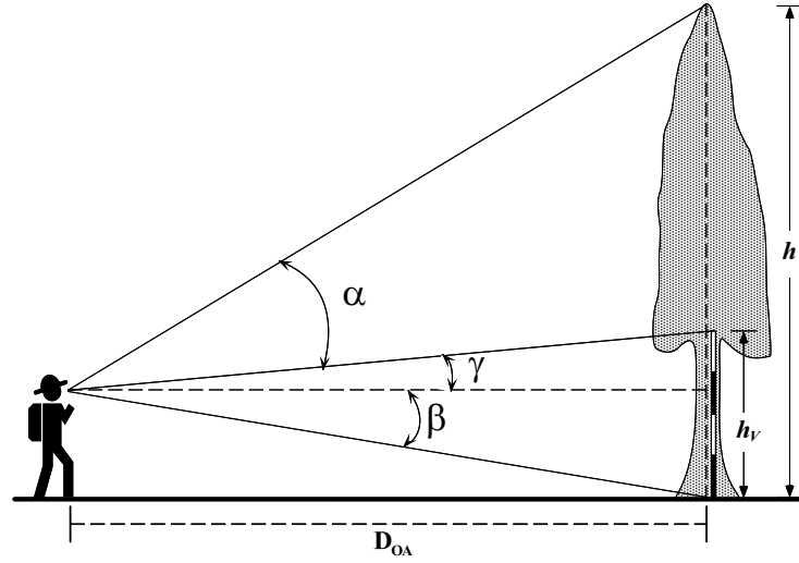
Figura 4.9: Aplicação da idéia do hipsômetro de Christen na medição da altura de árvores pelo método trigonométrico sem o conhecimento da distância observador-árvore.
