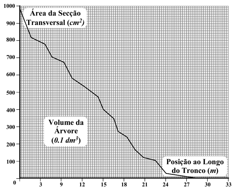
Figura 5.7: Cubagem de árvore inteira utilizando o método gráfico. No eixo das ordenadas ( y ) coloca-se a área seccional obtida em diferentes posições do tronco. No eixo das abcissas ( x ) coloca-se a distância a partir da base do tronco. O volume da árvore é definido como a área abaixo da linha do gráfico. As áreas seccionais devem ser plotadas em cm^2 e a distância da base em m, assim, a unidade de medida do volume é 0.1 dm^3 .
