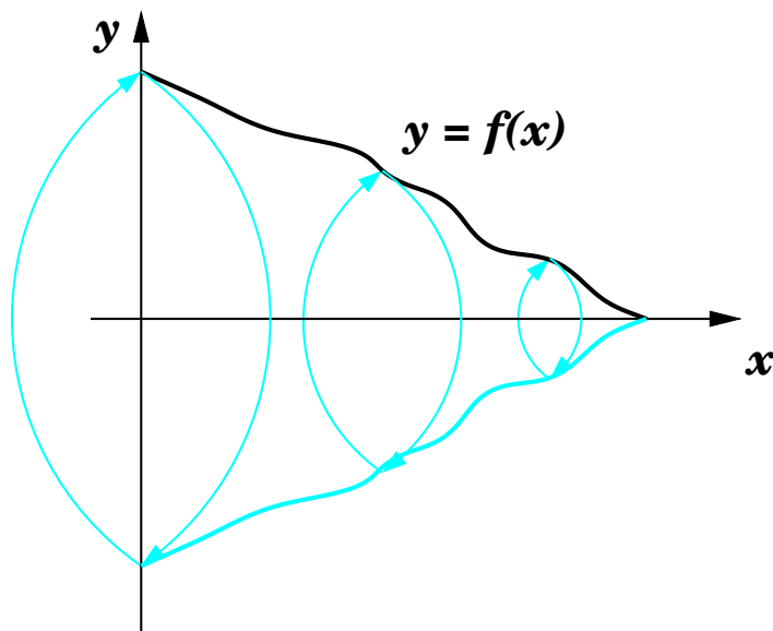
Figura 5.3: A rotação de uma função qualquer ( y = f(x) ) ao redor do eixo x (revolução) gera um sólido de base circular.
