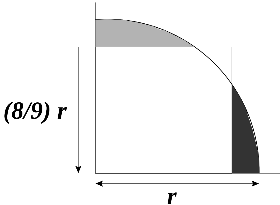
Figura 3.2: Esquema da aproximação utilizada no Egito Antigo para cálculo da área do círculo.
