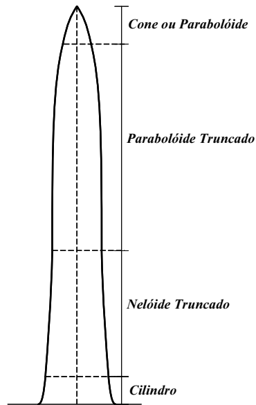
Figura 5.5: Variação da forma do tronco de acordo com a posição do torete (Husch et al., 1982).
