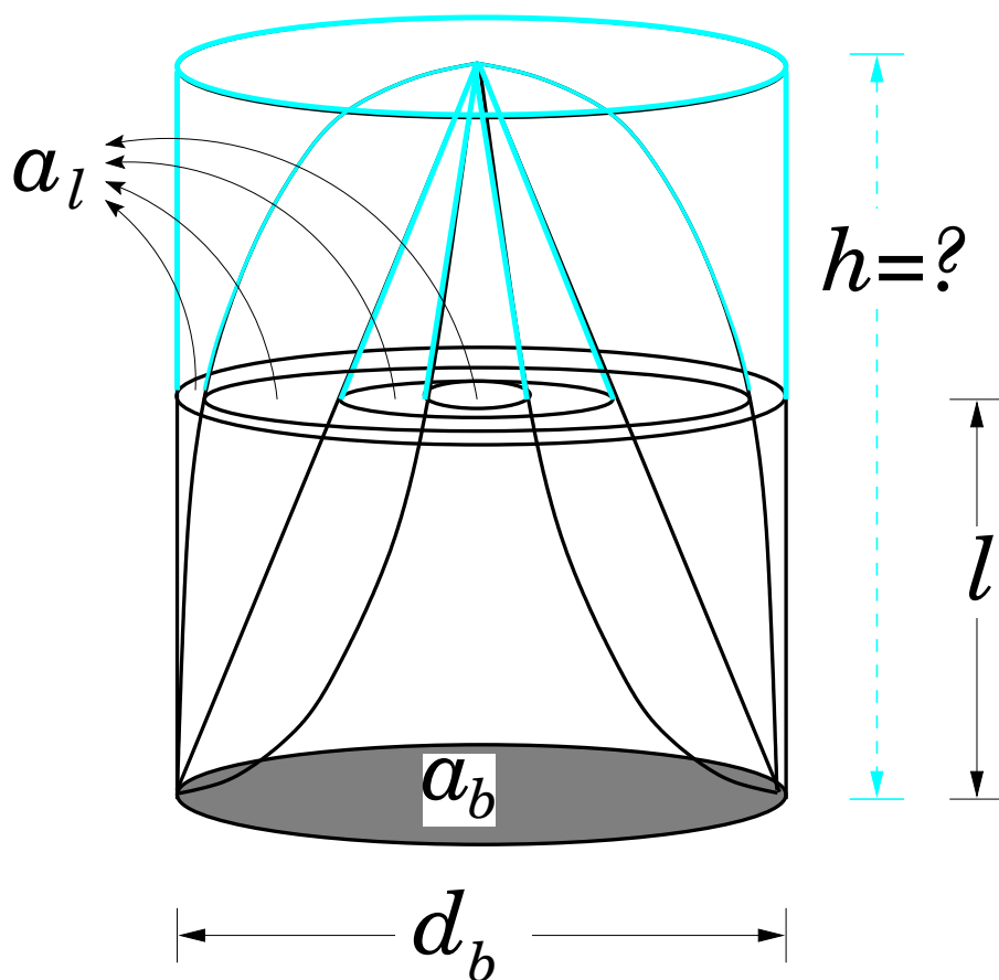
Figura B.1: Representação dos toretes do tronco de uma árvore através sólidos geométricos truncados. A altura total do sólido ( h ) é sempre desconhecida, mas é possível se medir o comprimento do torete ( l ) e obter as áreas das duas faces do torete (base: a_b e topo: a_l ) medindo-se os diâmetros.
