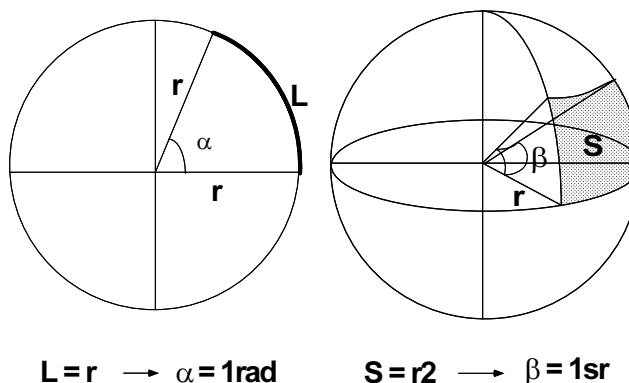
Figura 1.1: Medição de ângulos no plano e no espaço (3 dimensões) de acordo com o SI.
