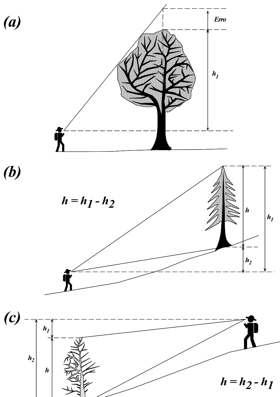
Figura 4.10: Problemas frequentes na medição de altura. Em (a), a visada muito próxima da árvore faz com que o observador confunda um ramo lateral como o ramo mais alto da árvore. Em (b) e (c), a medição em áreas muito declivosas faz com que as visadas do topo e da base da árvore estejam acima ou abaixo da linha horizontal que passa pela altura dos olhos do observador.
