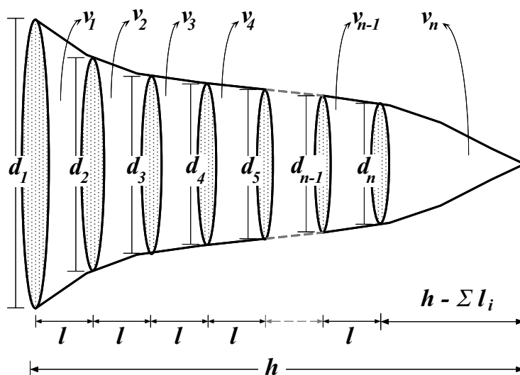
Figura 5.6: Cubagem rigorosa de árvore inteira com toretes de mesmo comprimento. O comprimento da ponta da árvore é a diferença entre a altura total e a somatória dos comprimentos ( h - \sum l_i ), e o volume da ponta é obtido assumindo que esta é perfeitamente cônica.
