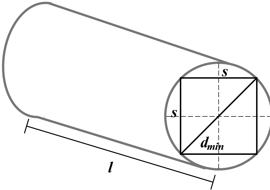
Figura 5.8: Método da Alfândega de Paris para a quantificação do volume útil para serraria em madeira roliça. O volume útil é definido como o sólido geométrico de base quadrada a partir do quadrado circunscrito na face de menor diâmetro da tora: s é o lado da base quadrada, d_{min} é o diâmetro da tora na sua menor face, sendo também a diagonal da base quadrada, e l o comprimento da tora.
