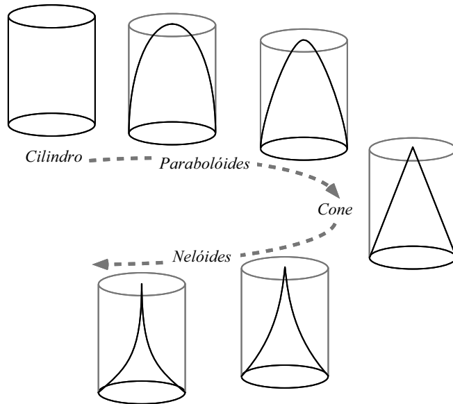
Figura 5.2: Exemplos de sólidos geométricos de base circular. Como resultado da mudança na forma do sólido, o volume decresce a partir do cilindro, embora a área da base e a altura permaneçam constantes.
