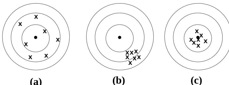
Figura 1.2: Representação gráfica dos conceitos de precisão, viés e exatidão, simulando o alvo de três atiradores diferentes. (a) apresenta um atirador com pequena precisão mas sem viés. Em (b) o atirador tem alta precisão mas apresenta um viés em relação ao centro do alvo. O alvo (c) é do atirador com precisão e sem viés, portanto, o atirador mais exato .
