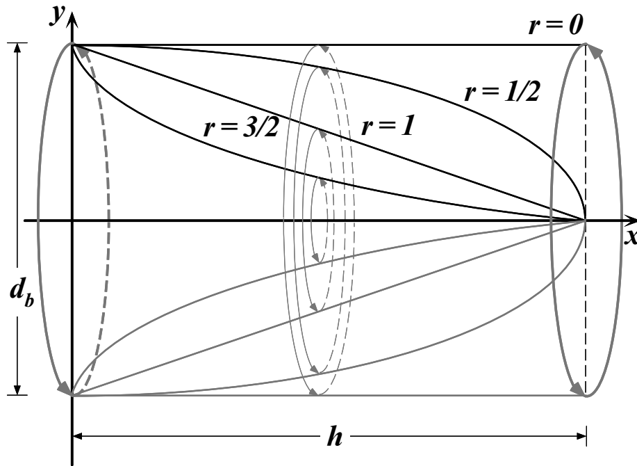
Figura 5.4: Formação dos sólidos geométricos da família do cilindro a partir da rotação de uma função no plano cartesiano x-y que represente a variação do raio ( y ) em função da altura ( x ) a partir da base. Duas medidas dos sólidos permanecem inalteradas: o diâmetro da base ( d_b ) e a altura total ( h ).
