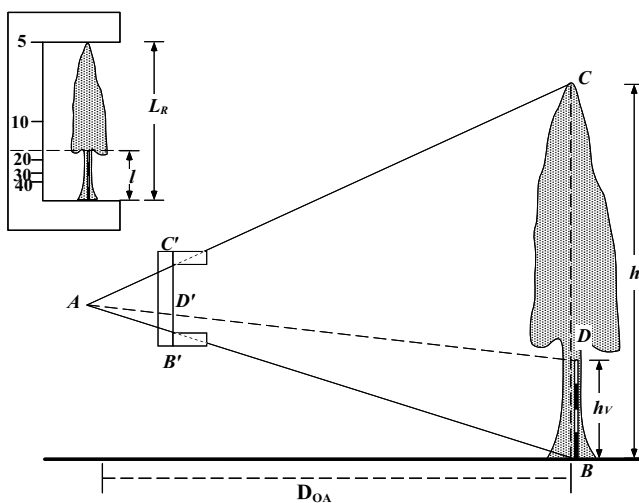
Figura 4.6: Funcionamento do hipsômetro de Christen, que utiliza uma régua para encaixe visual da árvore e uma baliza de altura conhecida. A fórmula deste hipsômetro é obtida com base em duas semelhanças de triângulos: entre os triângulos ABC e AB'C' e entre os triângulos ABD e AB'D' .
