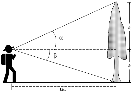
Figura 4.7: Funcionamento do método trigonométrico de medição de altura. Para as visadas de topo e base da árvore o instrumento mede o ângulo. Com o conhecimento da distância do observador à árvore e da tangente dos ângulos medidos, a altura da árvore é determinada.
