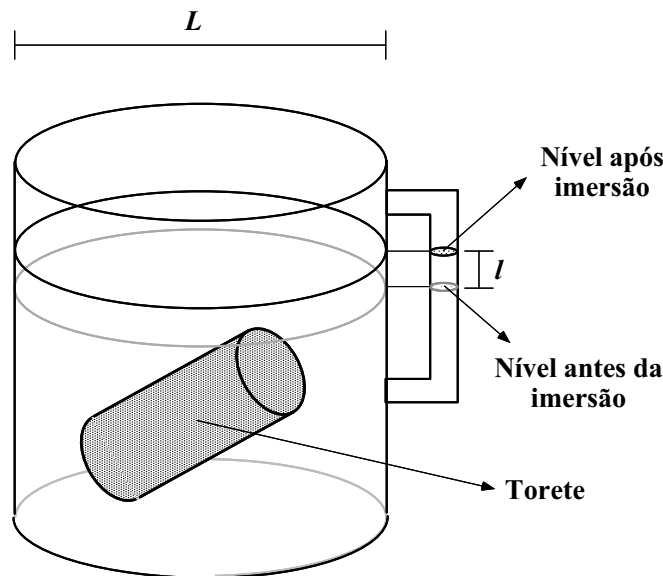
Figura 5.1: Utilização do Xilômetro para cubagem de toretes.
