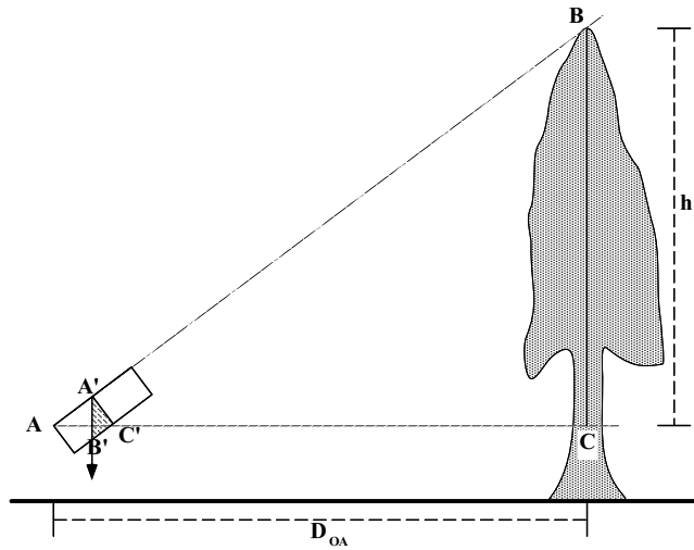
Figura 4.3: Funcionamento da prancheta dendrométrica quando é realizada uma visada do topo da árvore.
