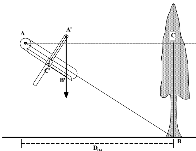
Figura 4.5: Funcionamento do hipsômetro de Weise. A semelhança de triângulos é a mesma que ocorre na prancheta dendrométrica, mas no hipsômetro de Weise a altura do pêndulo ( A'C' ) é ajustável.
