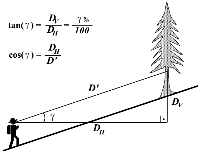
Figura 4.8: Efeito da declividade do terreno na medição da distância observador-árvore. \gamma é o ângulo de declividade do terreno, D' é a distância sobre o terreno D_H é a distância horizontal e D_V é o deslocamento vertical provocado pela declividade.
